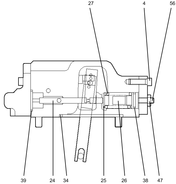
B-B KESİTİ SECTION B-B
