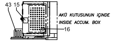
AKÜ KUTUSU ÜST GÖRÜNÜŞÜ ACCUM. BOX / UPPER VIEW
